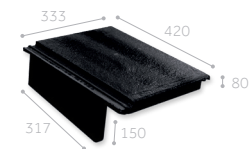
Telha de ventilação
